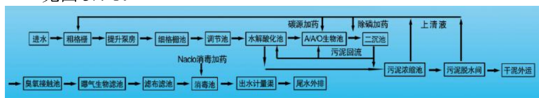
图 3.4-1 水处理工艺流程及产污节点图
